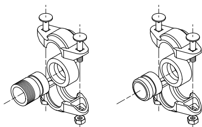
Fig. 16 PJE couplings
